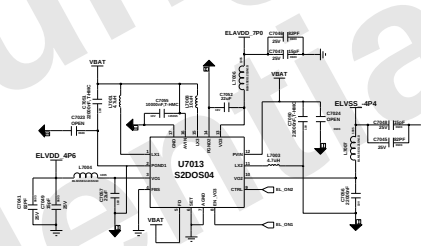
HD OCTA DC-DC
